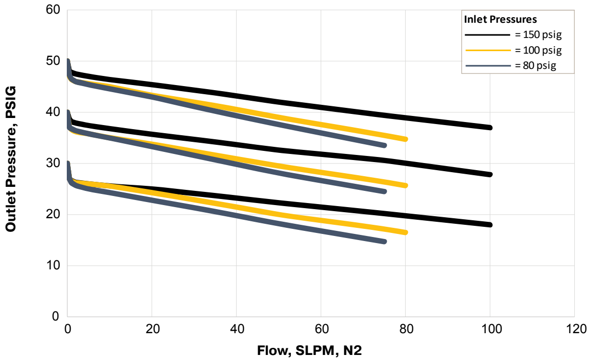
FR1000/FRN1000 — .09 Cv
