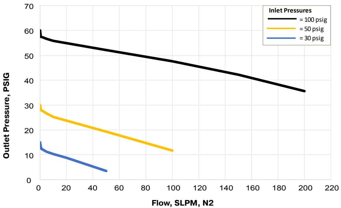
FR1000/FRN1000 — .15 Cv
